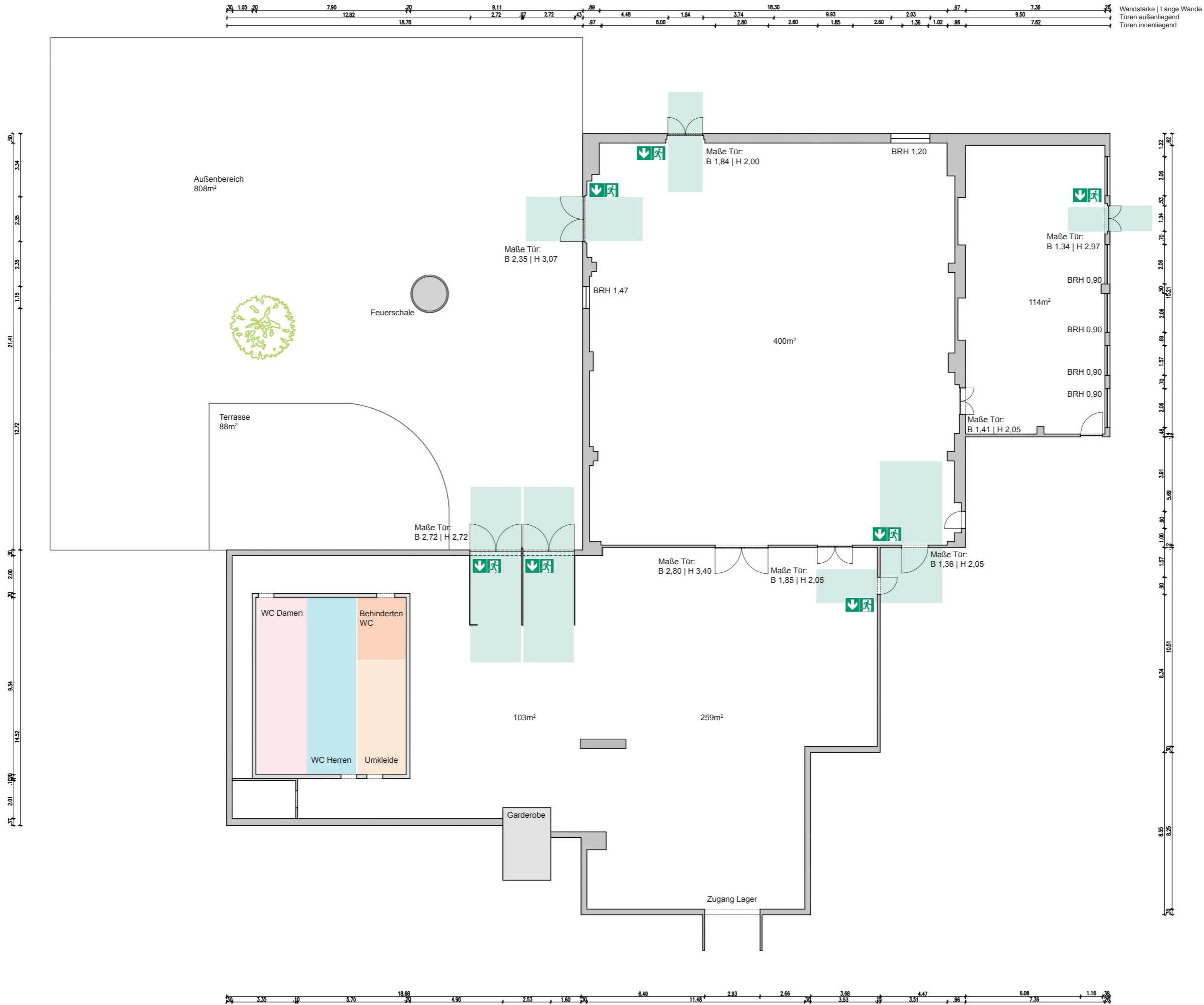
Grundriss Kulturbetrieb Wagenhallen Maßstab: 1:200 Mauerwerk Notausgang Freifläche Notausgang
